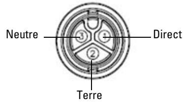
Illustration 8 Connecteur du câble d'alimentation c.a.
