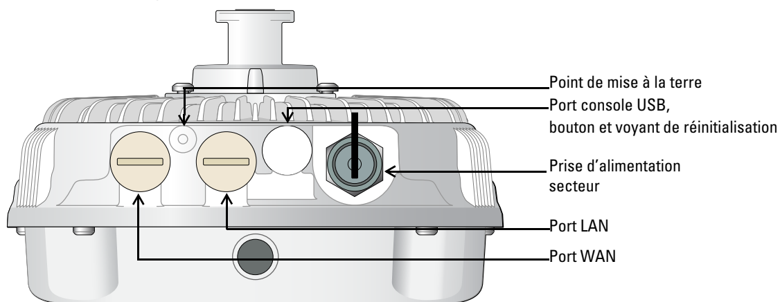
Illustration 2 Vue arrière du point d'accès W-IAP277
