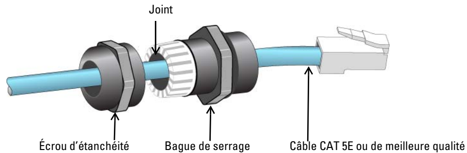
Illustration 7 Installation d'un presse-étoupe
