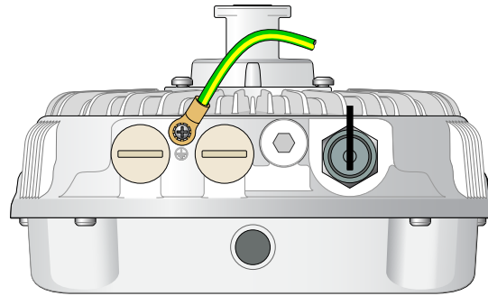
Illustration 6 Mise à la terre du point d'accès Instant
